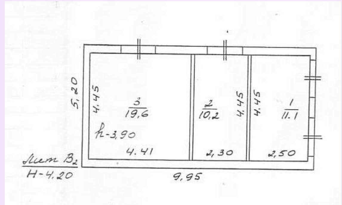
Здание трансформаторной подстанции
