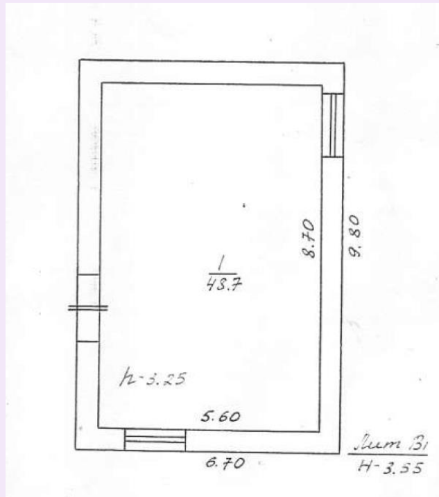
Здание дизельной электростанции
