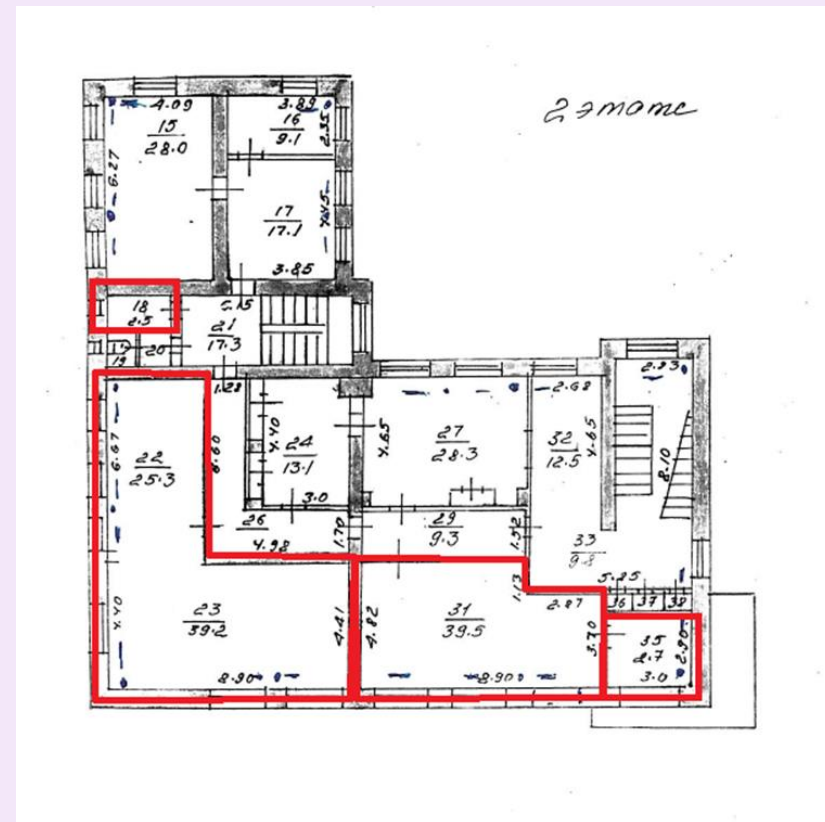
2 этаж
