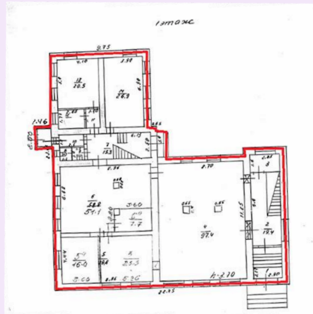
1 этаж
