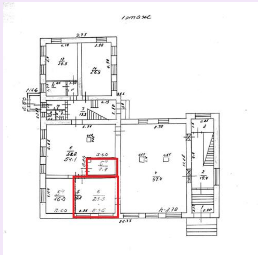
1 этаж
